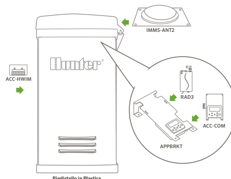
Installazione delle comunicazioni in ACC piedistallo
