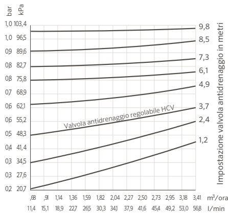
VALVOLA ANTIDRENAGGIO REGOLABILE HCV
